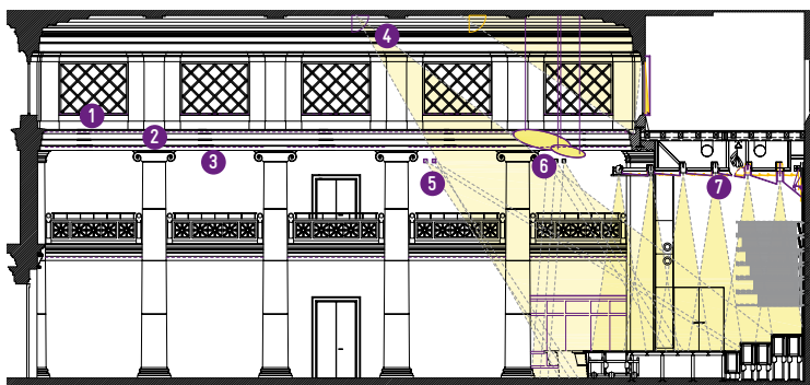
^Längsschnitt durch den Saal.
